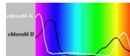
Ljusabsorption för två olika sorter klorofyll
